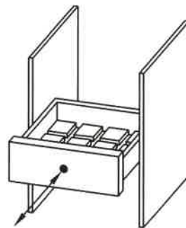
Схема испытания на долговечность
